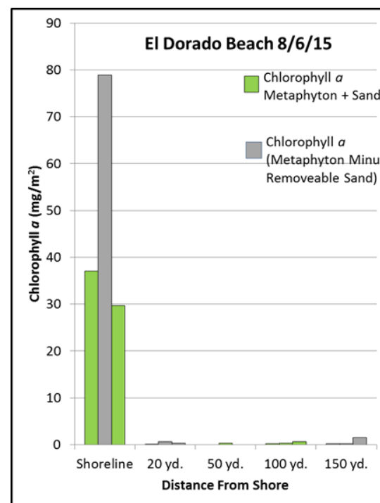
e. Metaphyton Chlorophyll a
