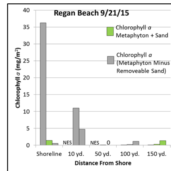
e. Metaphyton Chlorophyll a
